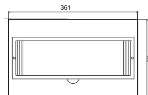
DB118/F 18 ways
