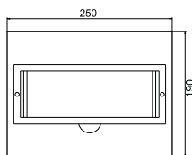
DB112/F 12 ways
